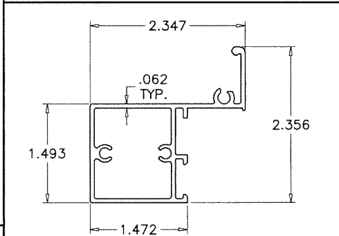
⑧ JAMB STILE
